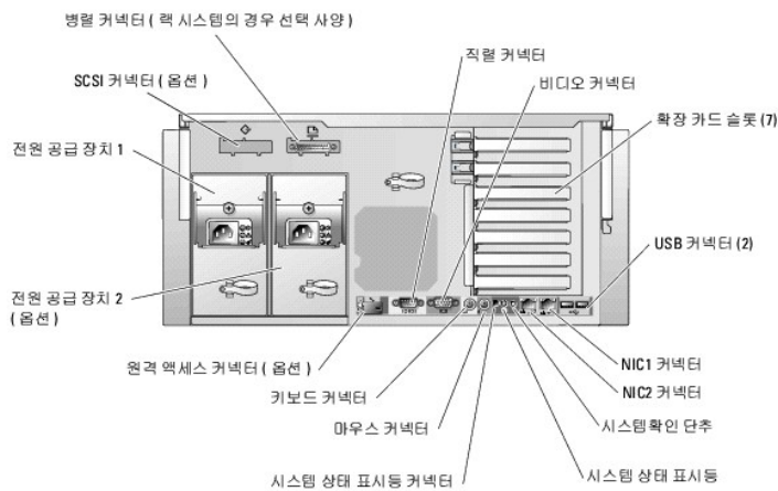
그림 1-4. 후면 패널 구조 및 표시등
