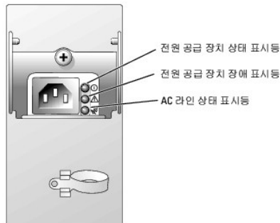
그림 1-5. 중복 전원 공급 장치 표시등
